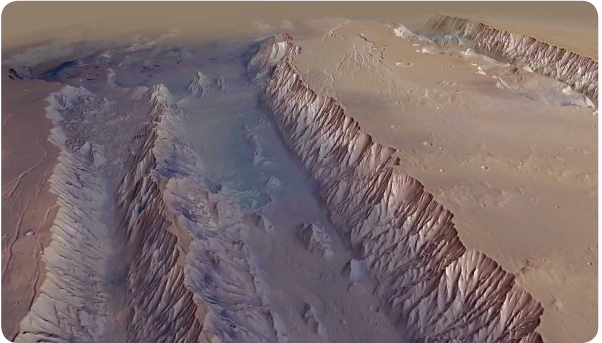
3D-Aufnahme der Valles Marineris, der größten Kraterlandschaft auf dem Mars.
